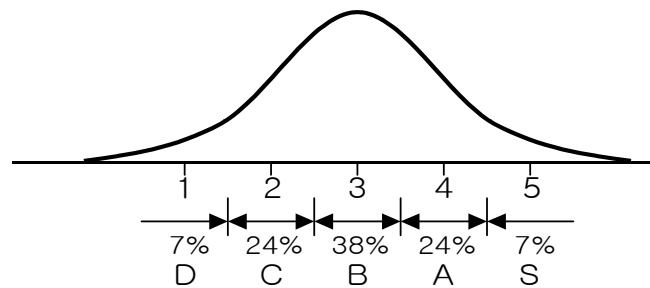
[그림 4] 표준 정규분포도
